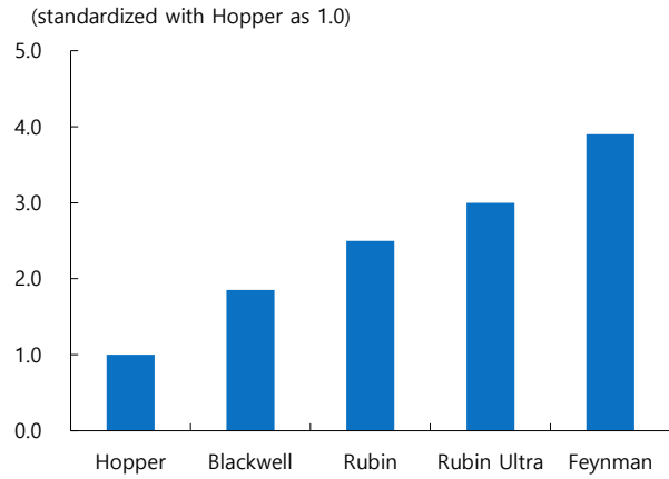
그림3. Nvidia GPU 세대별 substrate 소요량 비교
